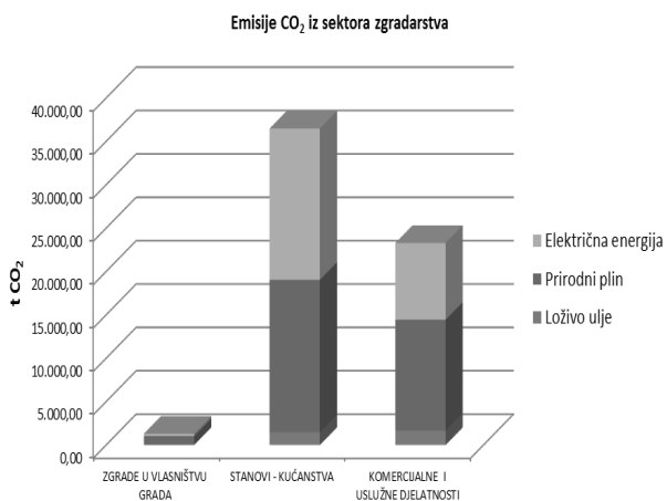
Slika 3. Emisije CO 2 iz sektora zgradarstva Grada Vinkovaca
